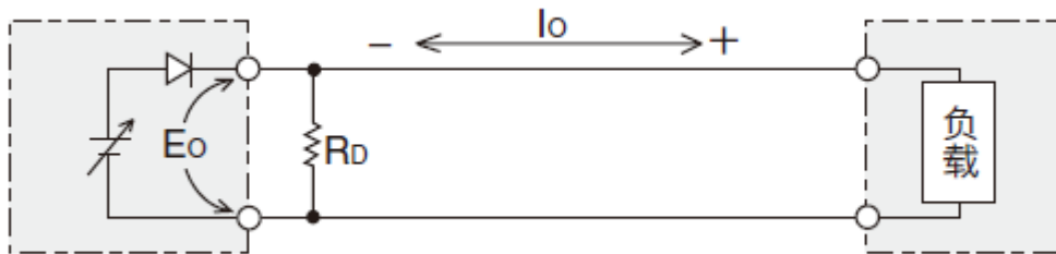
本产品的等效电路
