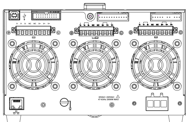
三通道机型:UDP5888H
