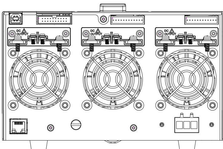
三通道机型:UDP5444/5888/5111/5222
