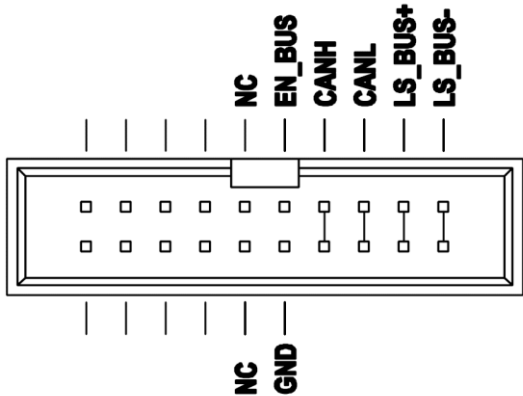
CAN 接口图
