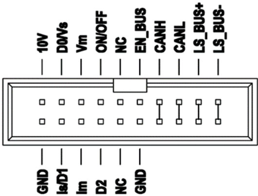
通道一外部接口
