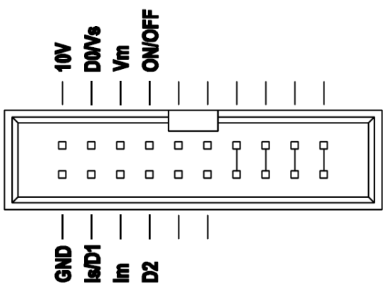
通道一外部接口
