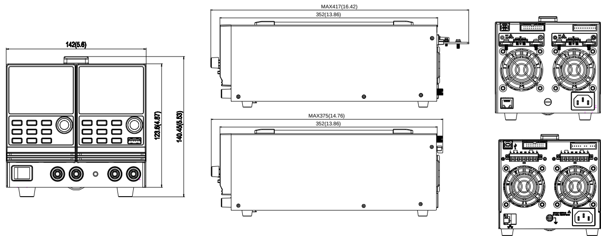
双通道机型:UDP5044,5088,5011,5022,5088H
