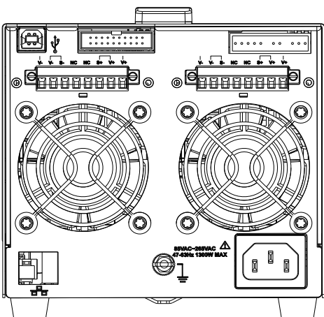
双通道机型:UDP5088H
