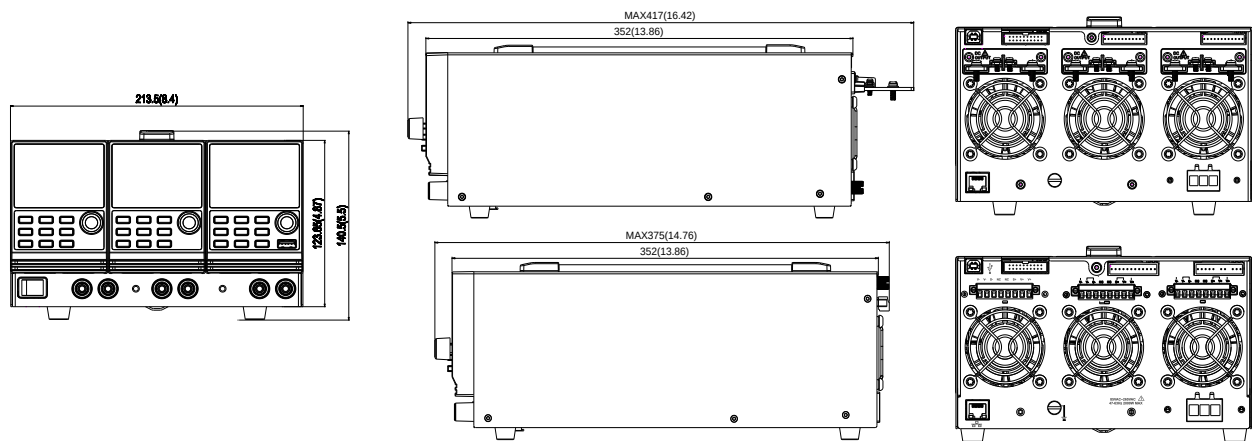
三通道机型:UDP5444,5888,5111,5222,5888H
