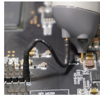
直角接地导线
